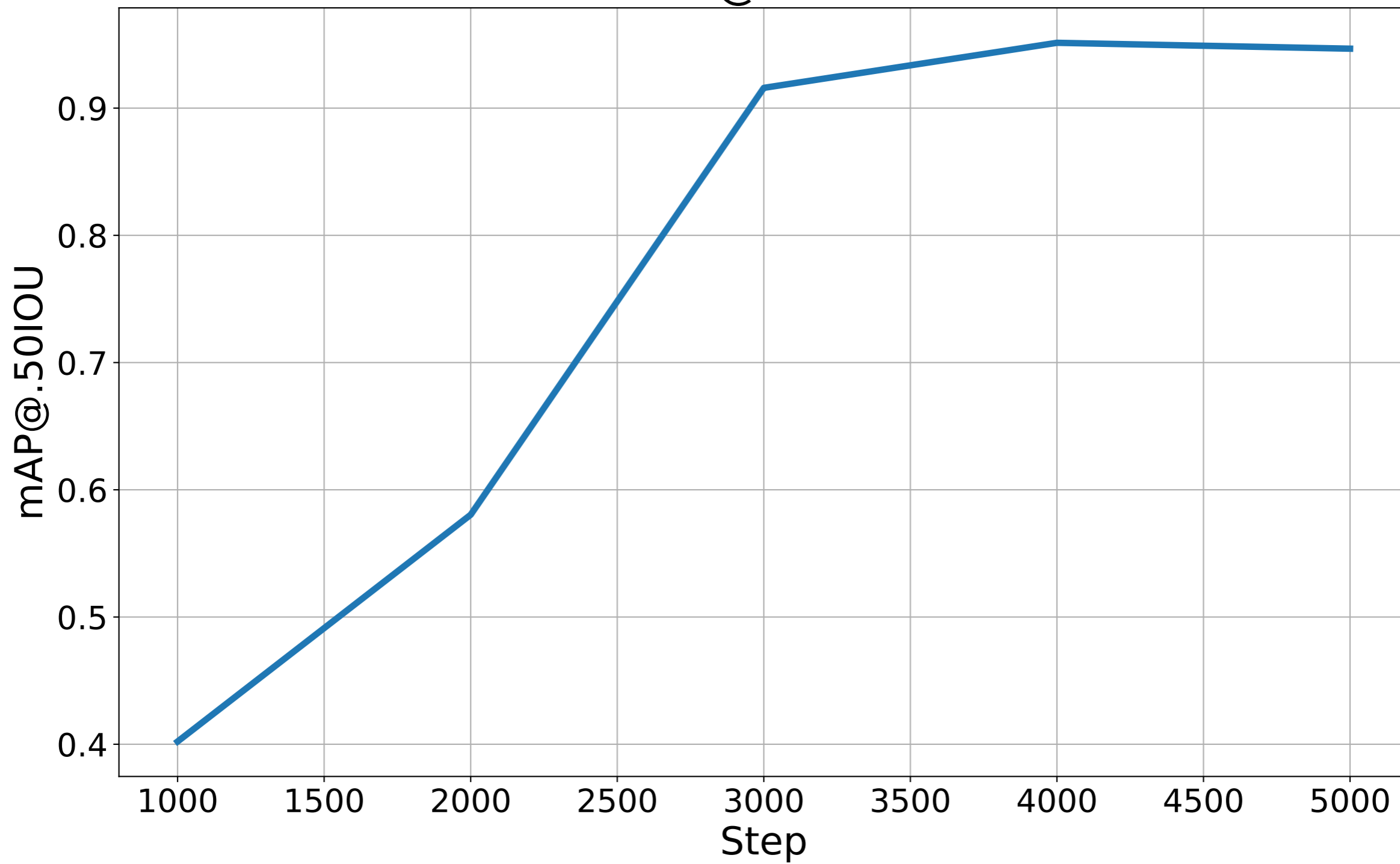
mAP@.50IOU
